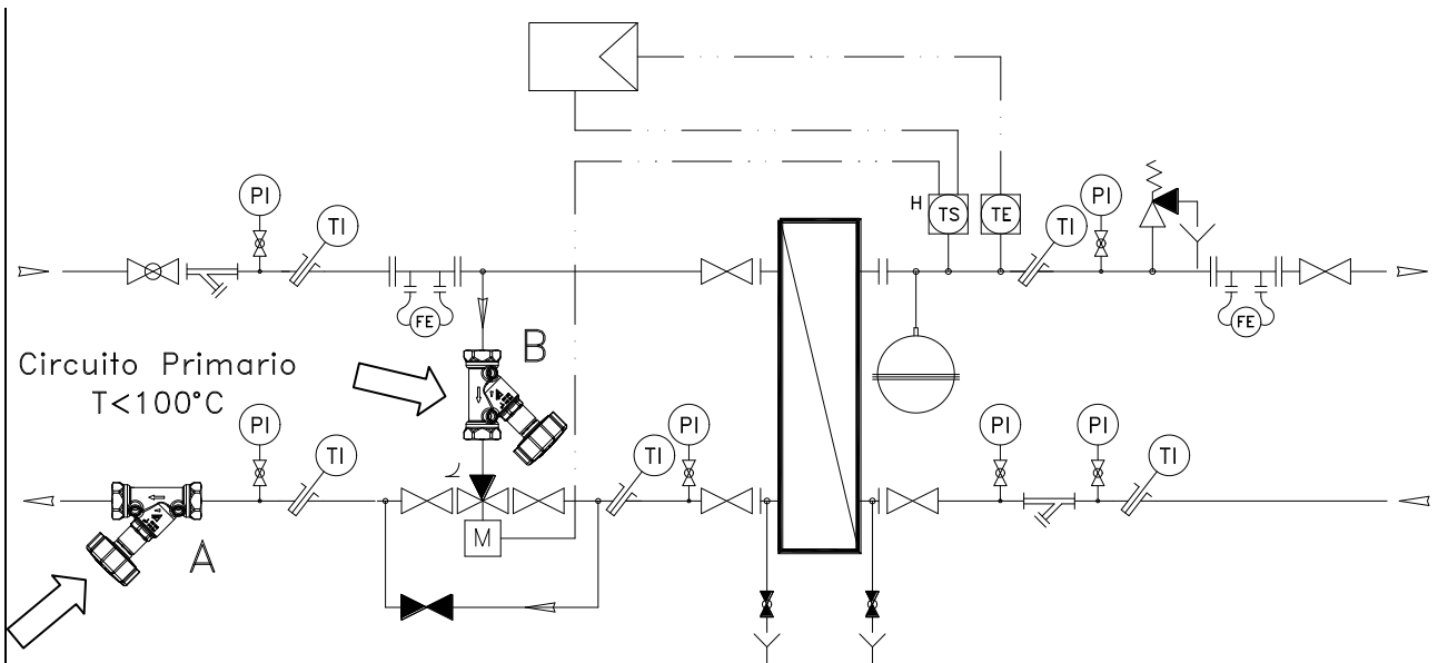
Schema 2 – Applicazione a sottocentrale di teleriscaldamento ad acqua calda.
