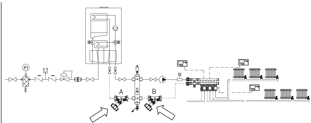
Schema 3 - Impianto di riscaldamento unifamilare.
