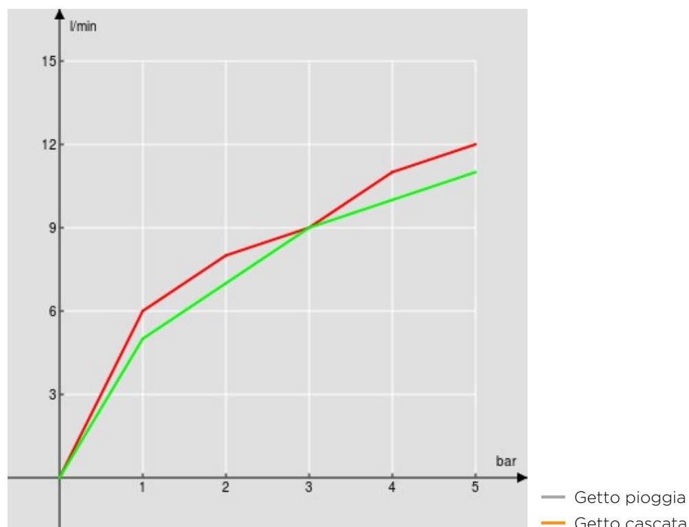
DIAGRAMMA DI PORTATA: ACQUA CALDA/FREDDA
