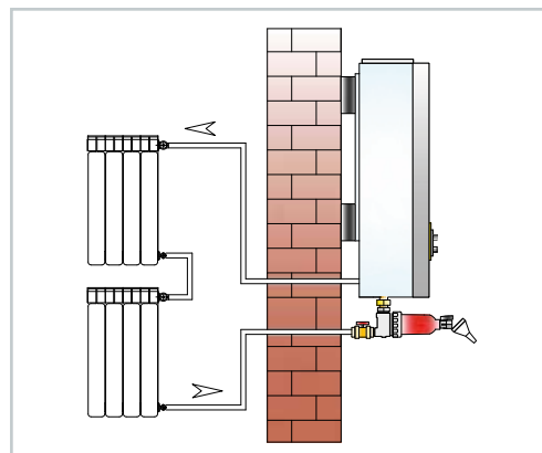
INSTALLAZIONE II
