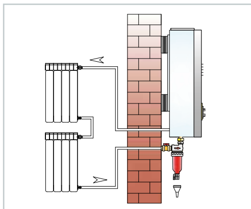
INSTALLAZIONE I
