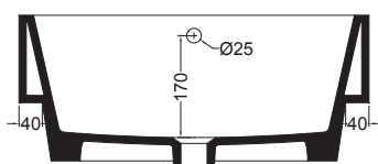
SEZIONE A-A
