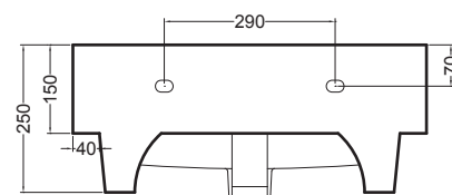
VISTA POSTERIORE
