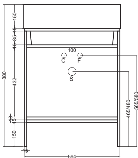
VISTA FRONTALE
