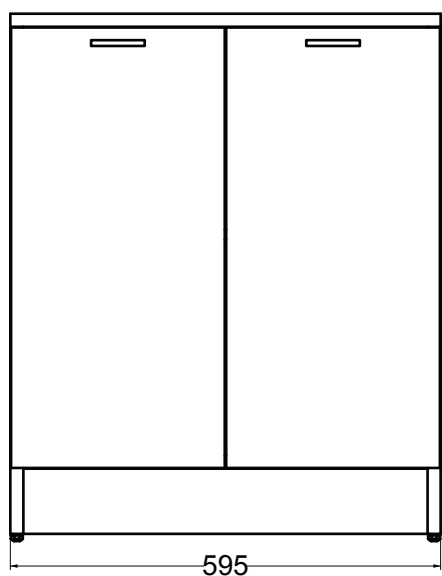
VISTA FRONTALE
