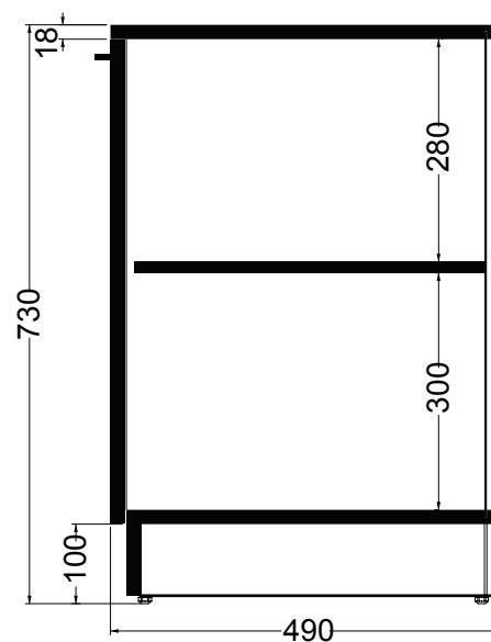
SEZIONE A-A
