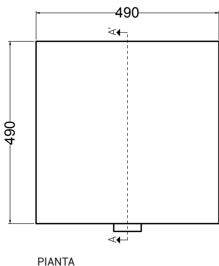
PIANTA
