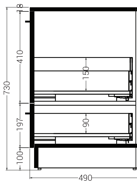
SEZIONE A-A
