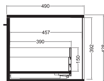
SEZIONE A-A
