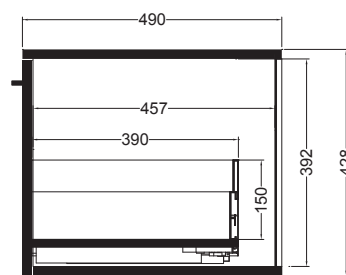
SEZIONE A-A
