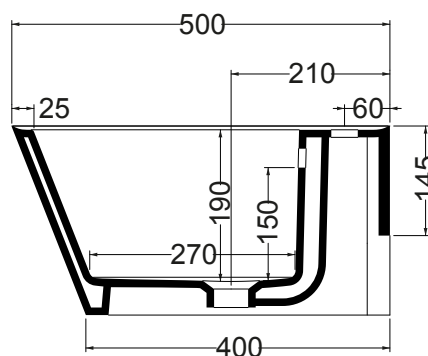
SEZIONE A-A'
