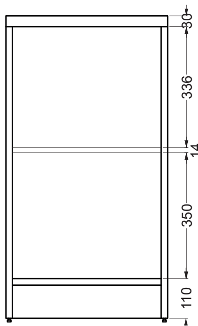
VISTA FRONTALE SENZA ANTA
